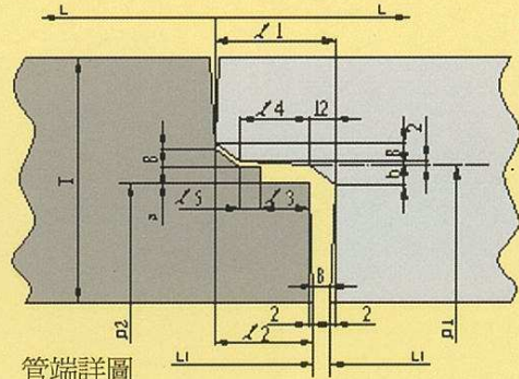
管端詳圖 detail for pipe end
