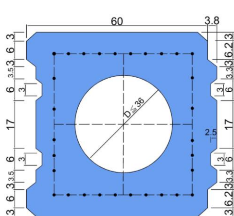
A-A 剖面圖
