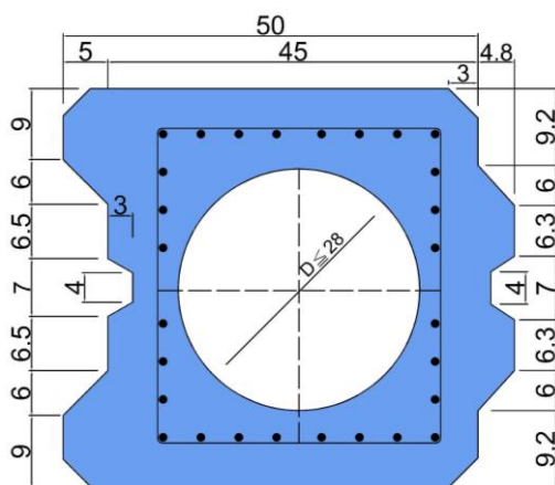
A-A 剖面圖
