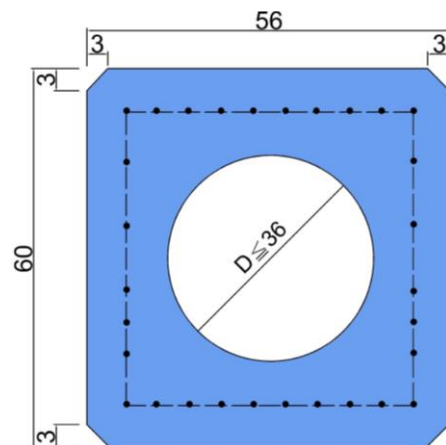
B-B 剖面圖
